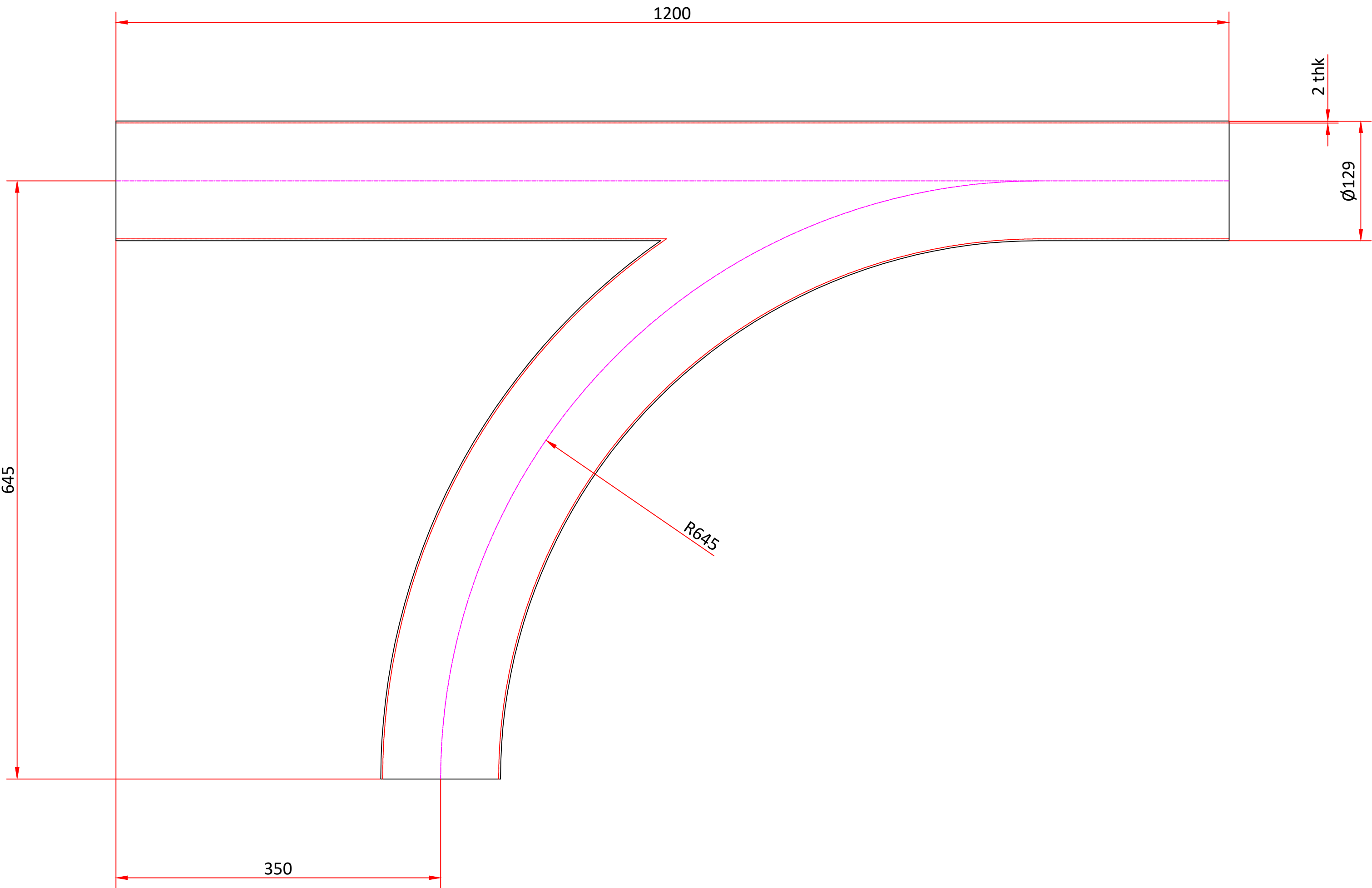
5" SWEPT TEE
